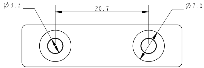
SCALE 2:1
