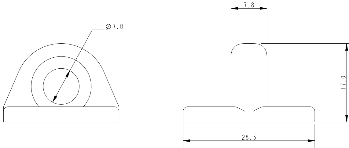
SCALE 2:1
