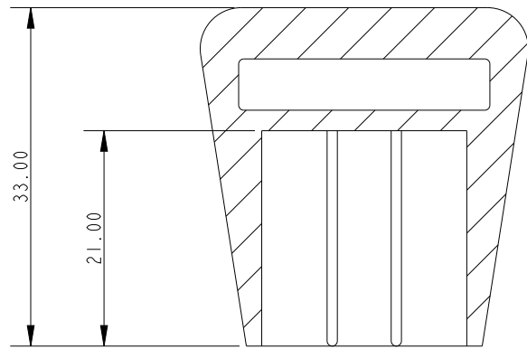
SECTION XSEC0001-XSEC0001 SCALE 3:2
