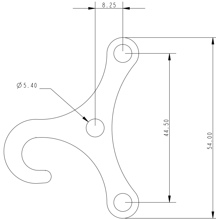
SCALE 3:2
