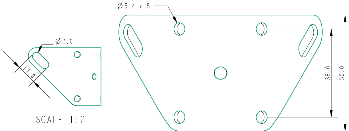
SCALE 1:1
