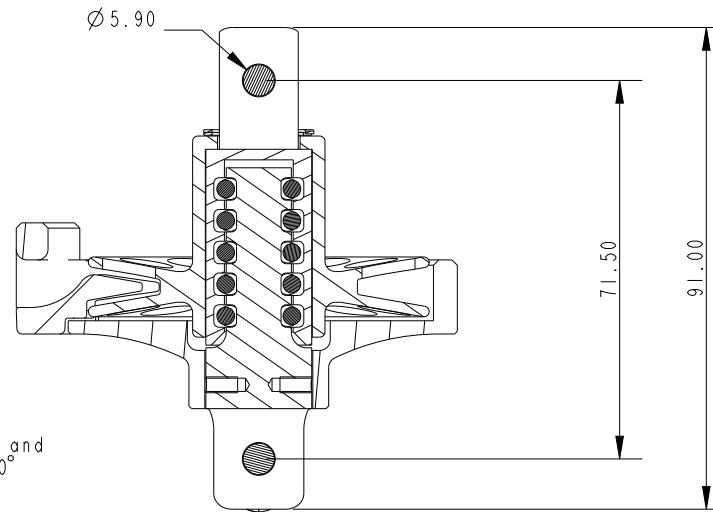
SECTION XSEC0001-XSEC0001
