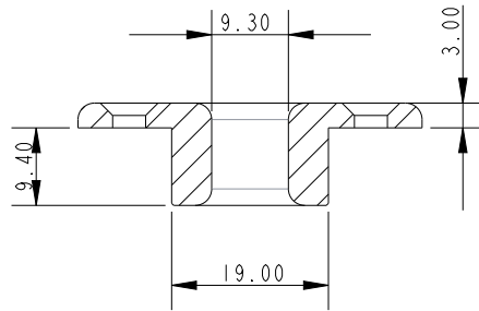
SECTION XSEC0001-XSEC0001
