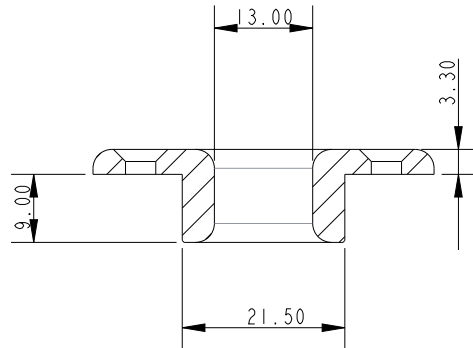
SECTION XSEC0001-XSEC0001
