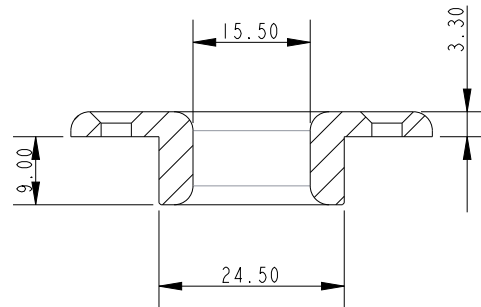
SECTION XSEC0001-XSEC0001
