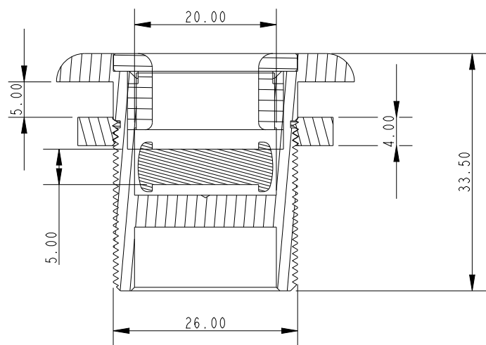
SECTION A-A SCALE 4:3
