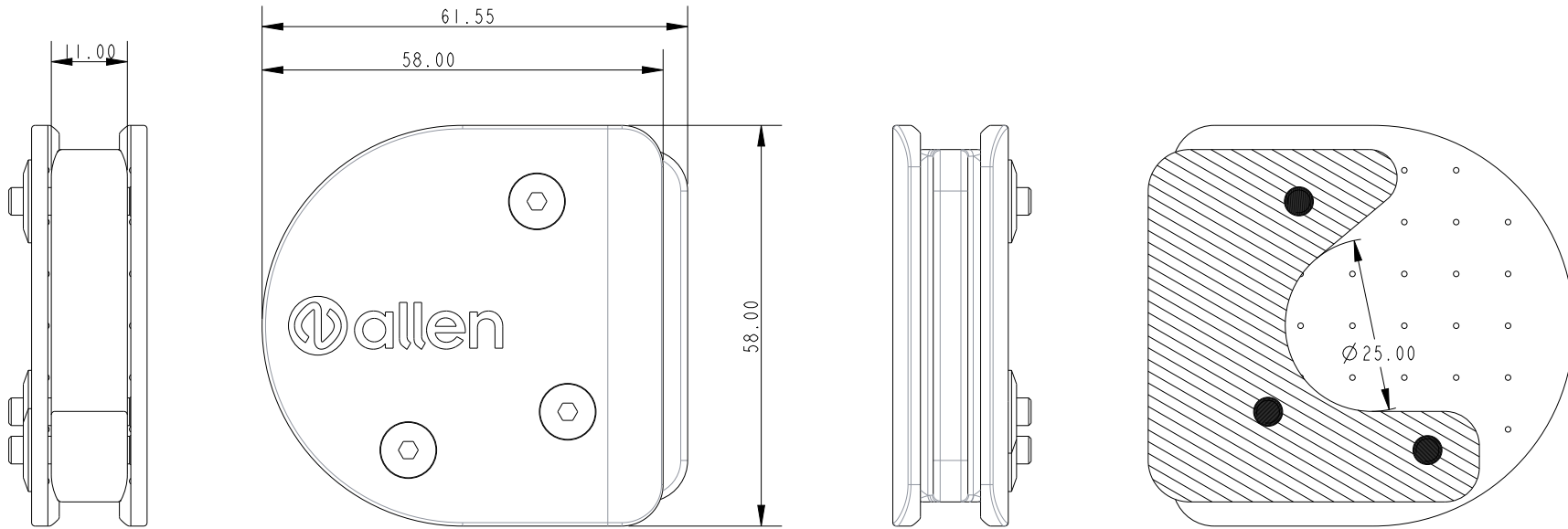
SECTION XSEC0001-XSEC0001
